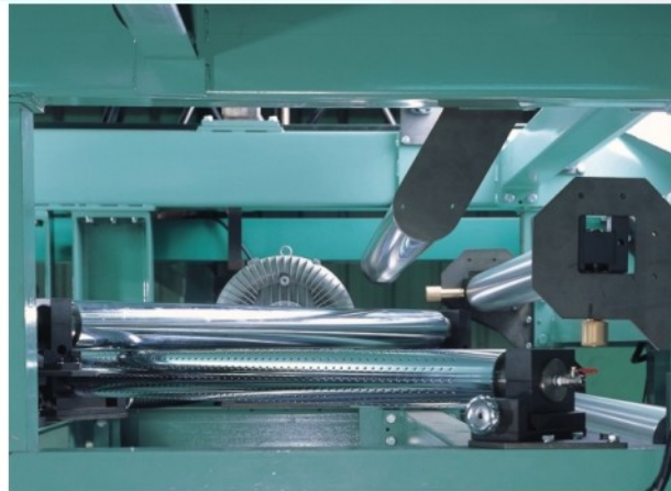
With 6+6 half web width turn bar 配備 6+6 半幅寬反轉架
